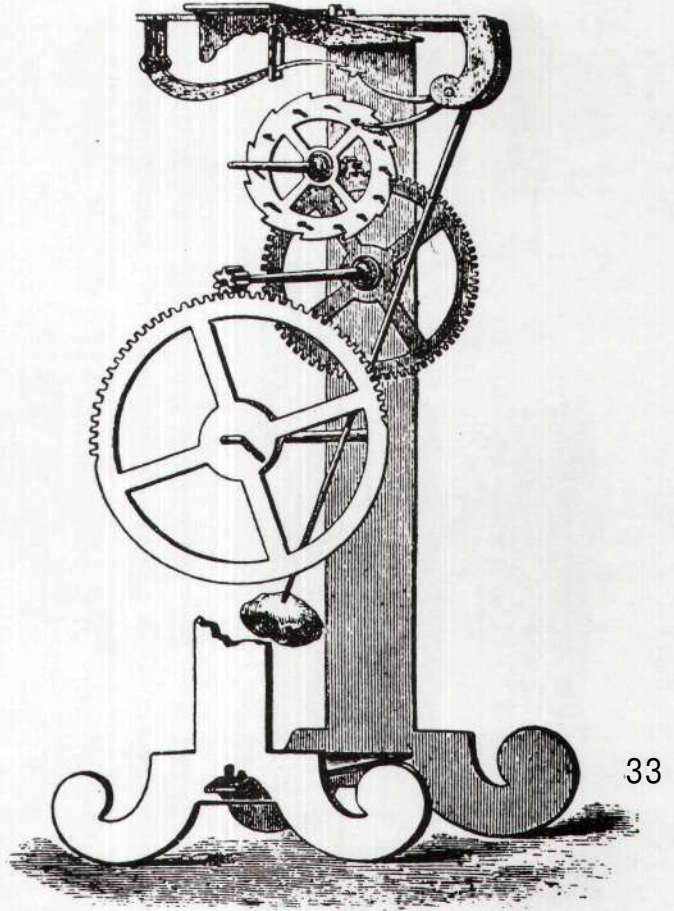
Galileo 'nun geliştirdiği sarkaçlı saat
