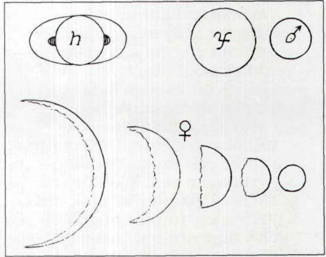
Galileo 'nun teleskobuyla gördüğü şekilleriyle gezegenler. En üstte soldan sırasıyla Satürn, Jüpiter ve Mars. Altta da Venüs'ün dönemlerinin çizimi.
